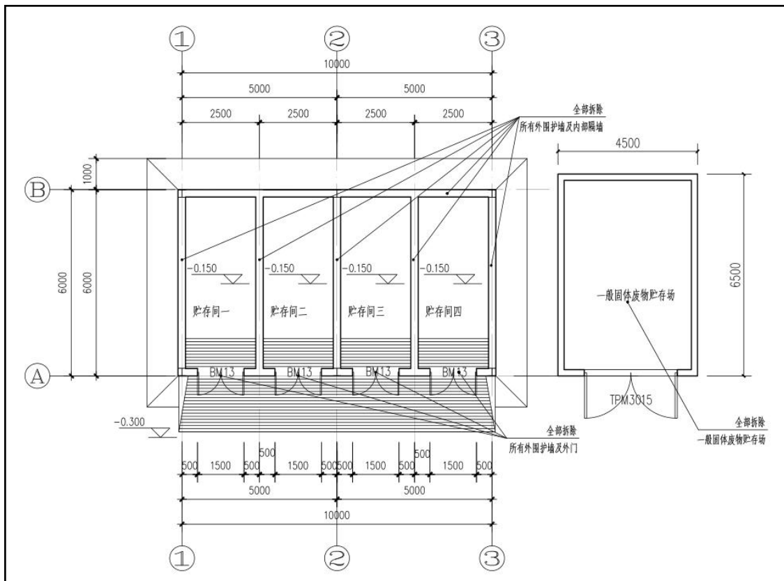
图 2-7 原有闲置库房平面布置示意图
