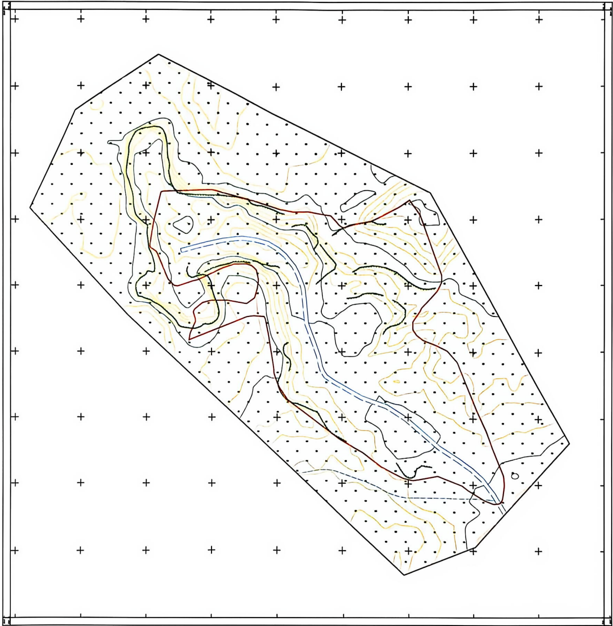
苏力德苏木塔来乌素嘎查废弃矿坑生态修复治理及土地复垦项目地形图
